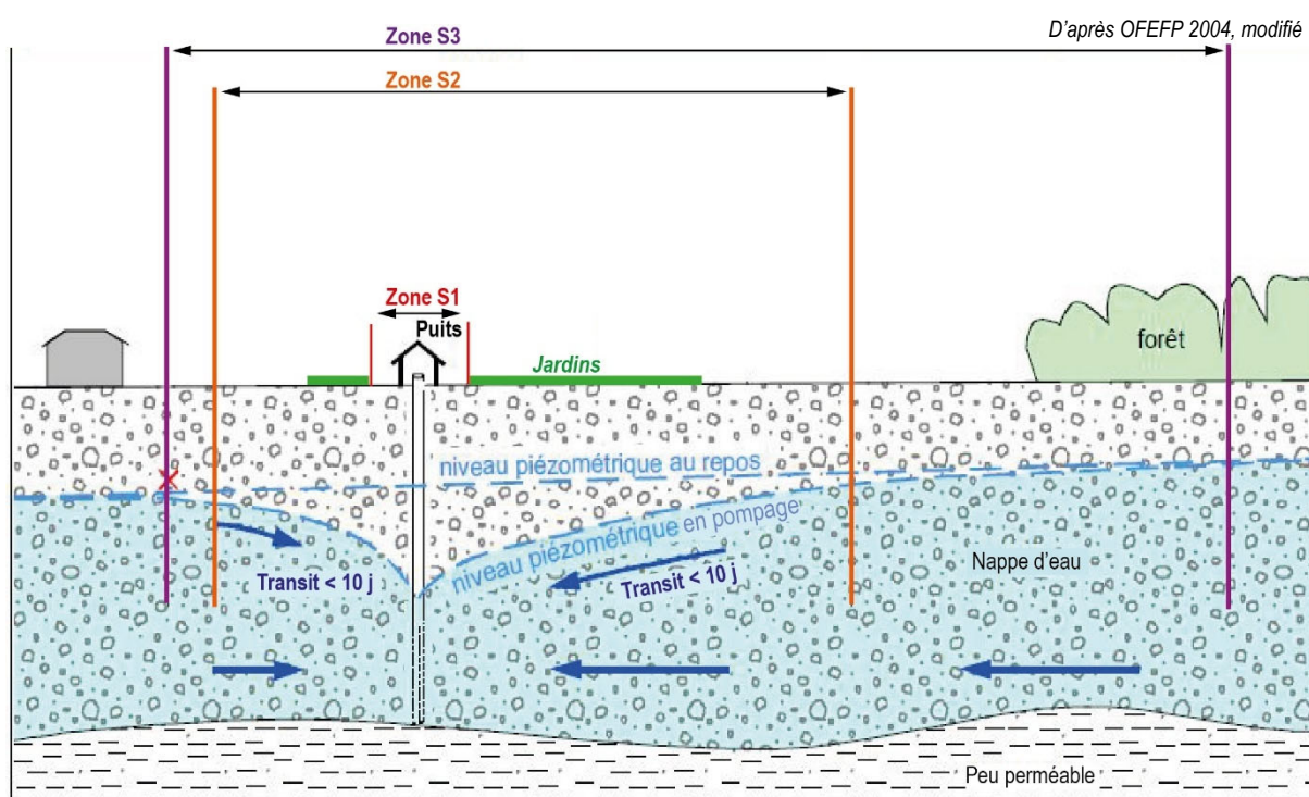
Schéma de principe de délimitation des zones de protection en plaine alluviale
