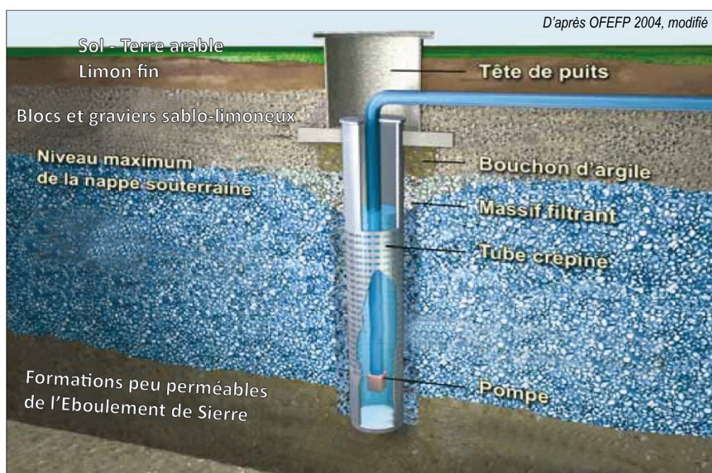
Coupe schématique d'un puits de captage – Contexte de la Raspille
